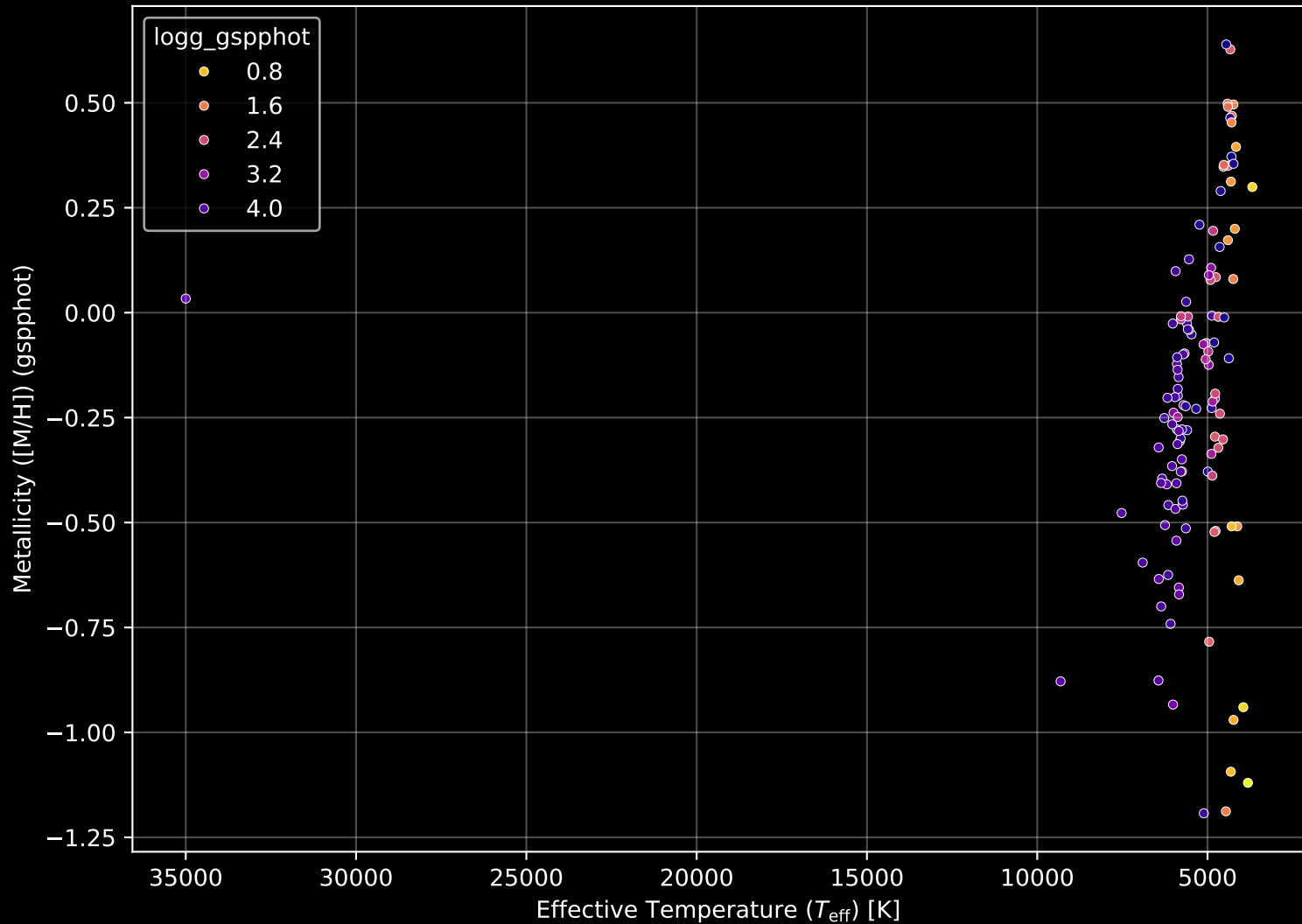
APOGEE DR17 Field: [282-34-O] Stellar Population Parameters (n= 123)
