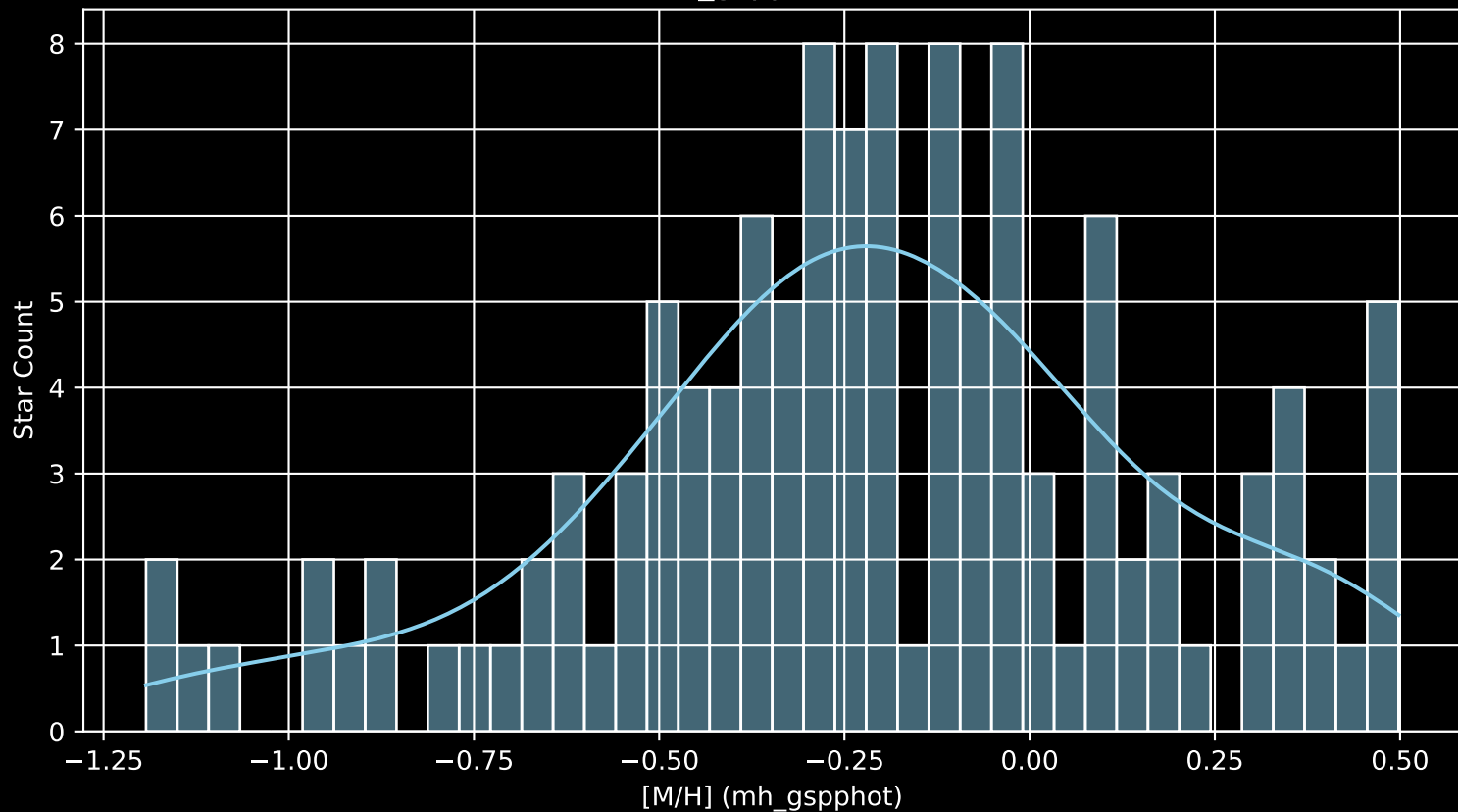
APOGEE DR17 Field: [282-34-O [M/H] (mh_gspphot) (n= 121)
