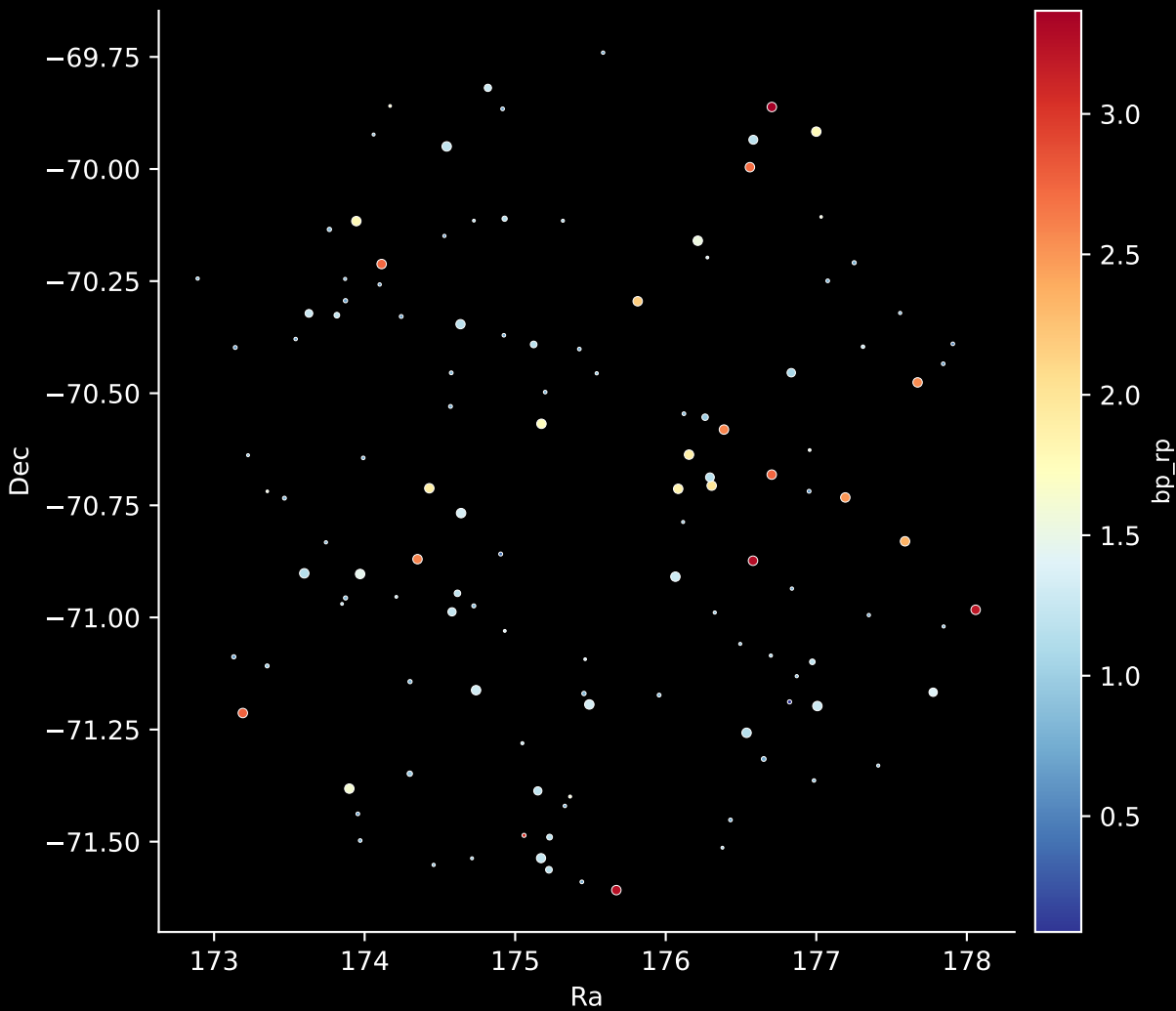
APOGEE DR17 Field: [282-34-O] Stars: 123
