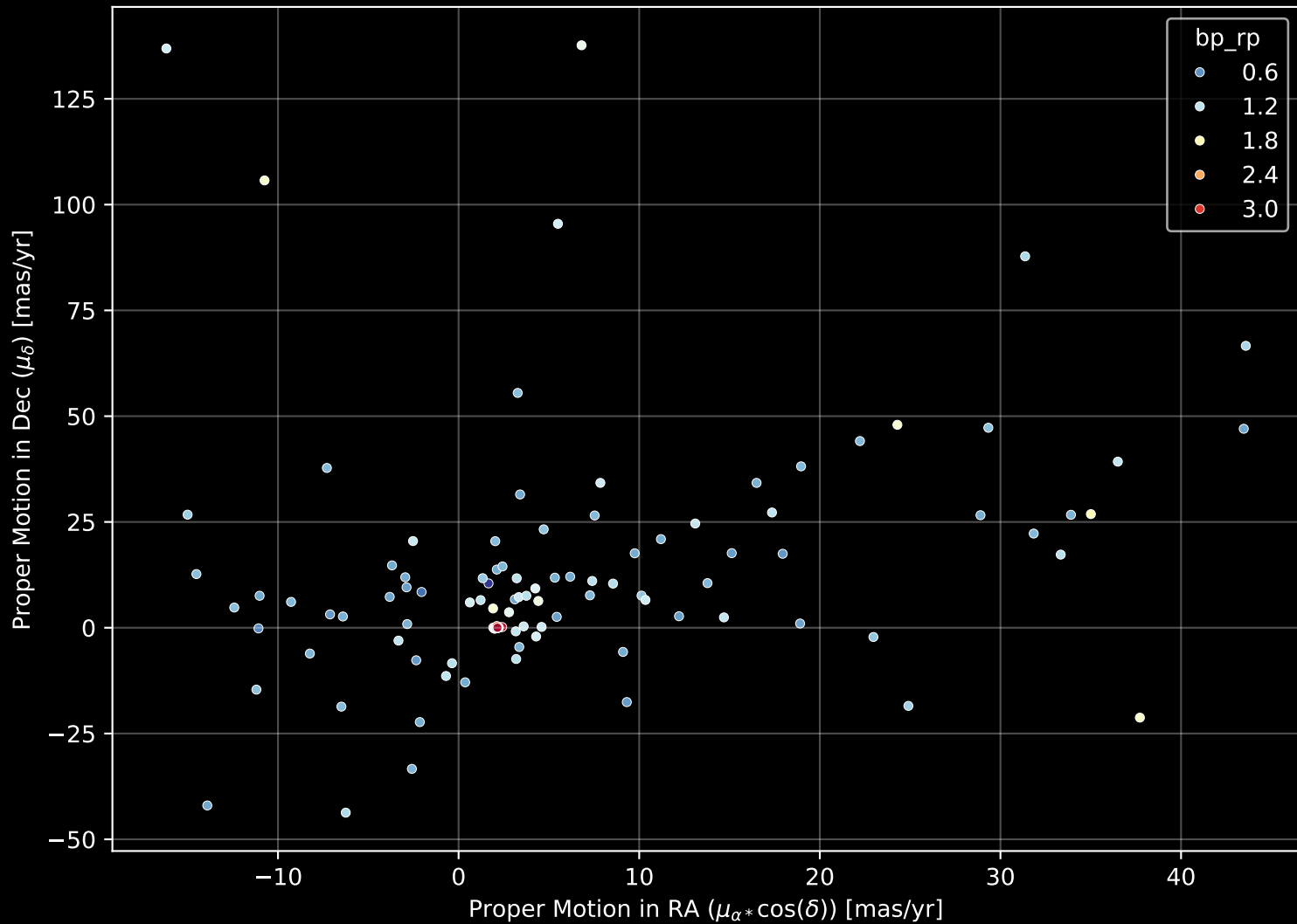
APOGEE DR17 Field: [282-34-O] Proper Motion Diagram (n= 123)
